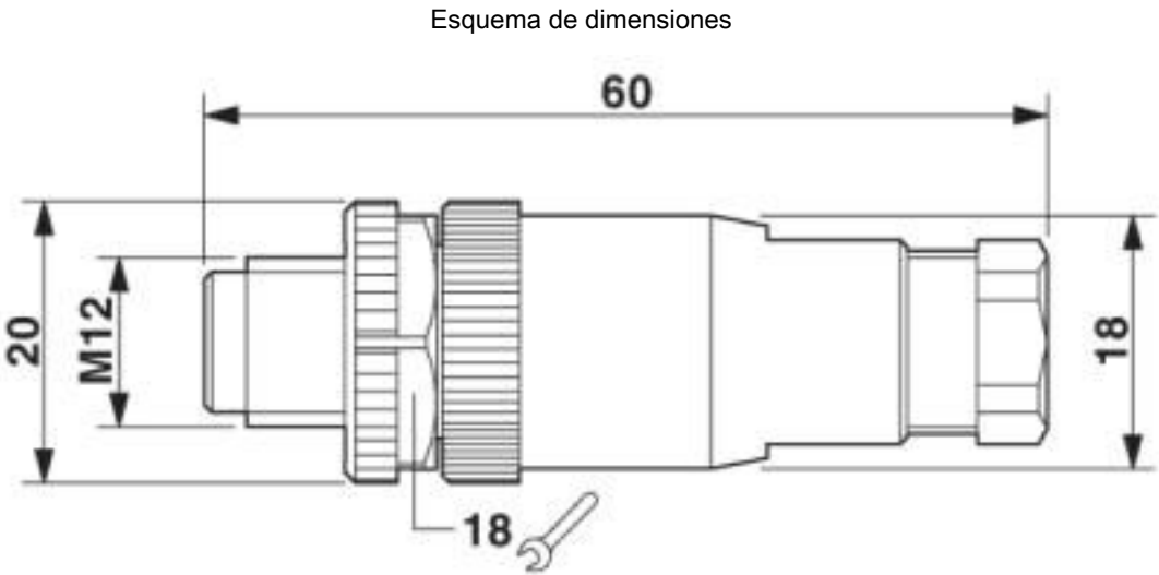
Conector macho M12 x 1, recto
